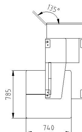
Draufsicht
